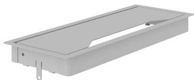
Metal grommet: 317x119 mm, H=27 mm
